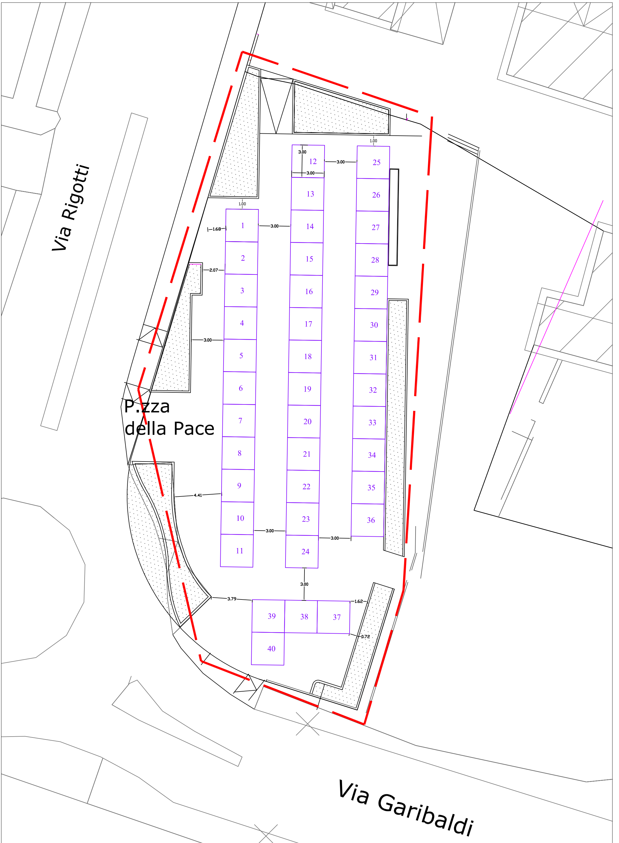
PLANIMETRIA OPERATORI NON PROFESSIONALI - scala 1:200
